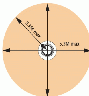
سطح پوشش آشکارساز حرارتی
