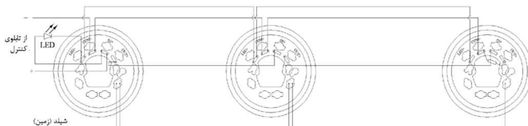
۳ آشکارساز با چراغ مشترک
