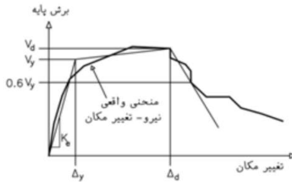
شکل ۲۳-الف-۵-۲ چند خطی کردن منحنی ظرفیت
