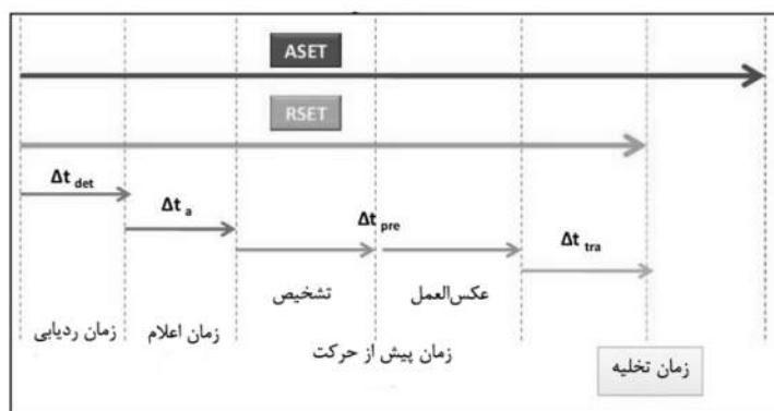
شکل ۲۳-ب-۴-۱: مثال مقایسه جدول زمانی بین ASET و زمان فرار
