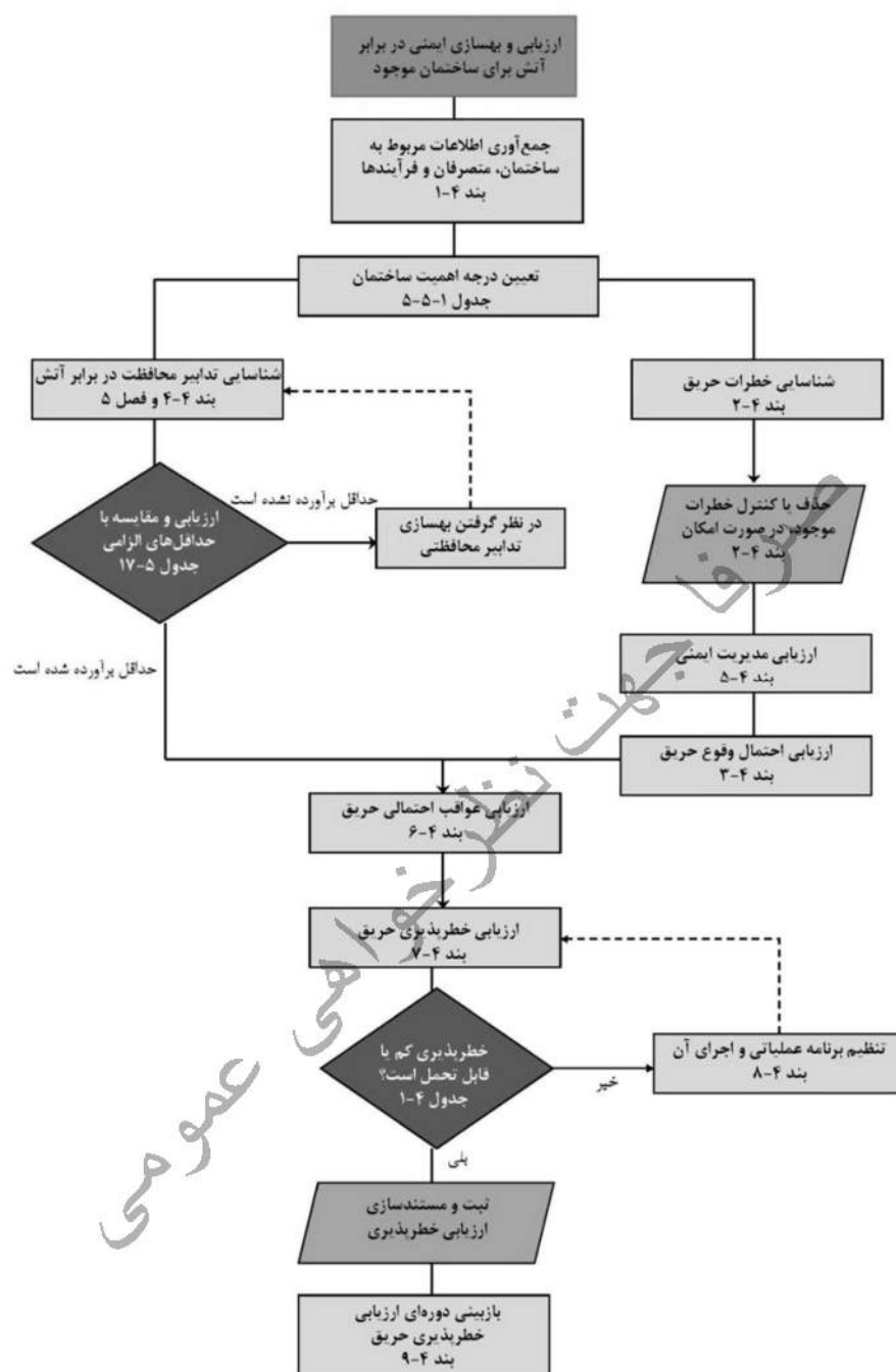
شکل ۲۳-ب-۳-۱: فلوچارت ارزیابی ایمنی در برابر آتش برای ساختمان‌های موجود
