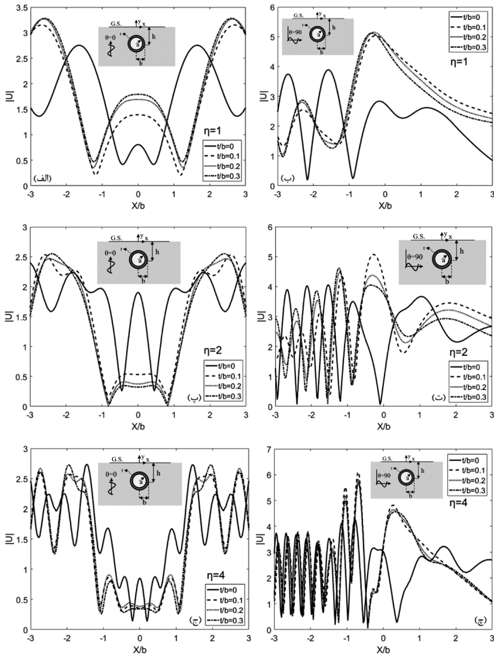
شکل (۷): دامنه تغییر مکان بی بعد شده سطح زمین در حضور تونل دایره ای پوشش دار مدفون در عمق 1.5h برای ضخامت های مختلف پوشش؛ (الف) \theta=0 , \eta=1 (ب) \theta=90 , \eta=1 (پ) \theta=0 , \eta=2 (ت) \theta=90 , \eta=2 (چ) \theta=0 , \eta=4 (ز) \theta=90 , \eta=4 .
