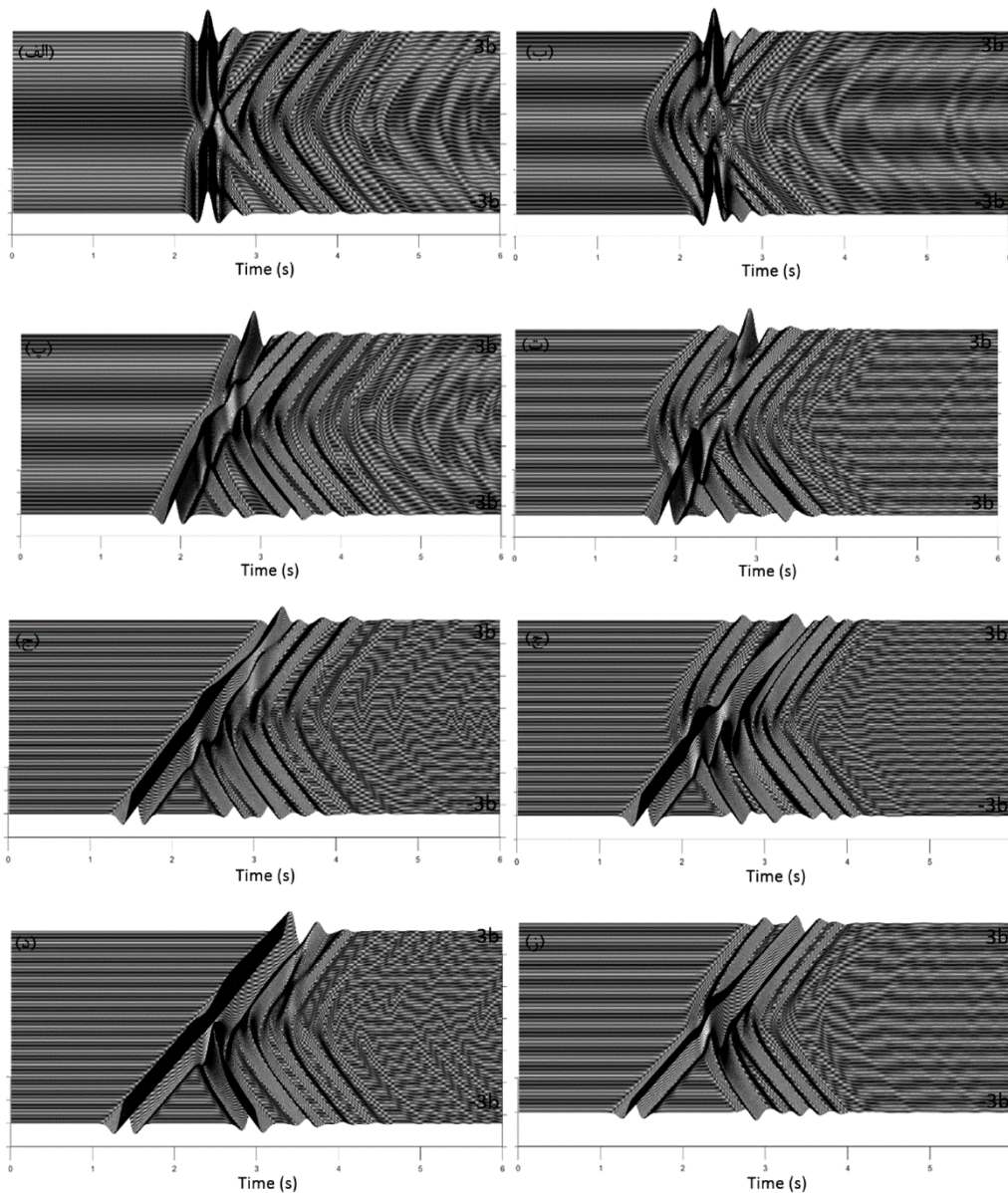
شکل (۴): پاسخ سطح زمین در حوزه زمان برای تونل دایره‌ای پوشش‌دار با ضخامت‌های متغیر 0 و 0.3b تحت تأثیر امواج مهاجم SH با زاویه \theta الف) t=0b, \theta=0 (ب) t=0.3b, \theta=0 (پ) t=0b, \theta=30 (ت) t=0.3b, \theta=30 (ج) t=0b, \theta=60 (چ) t=0.3b, \theta=60 (د) t=0b, \theta=90 (ز) t=0.3b, \theta=90
