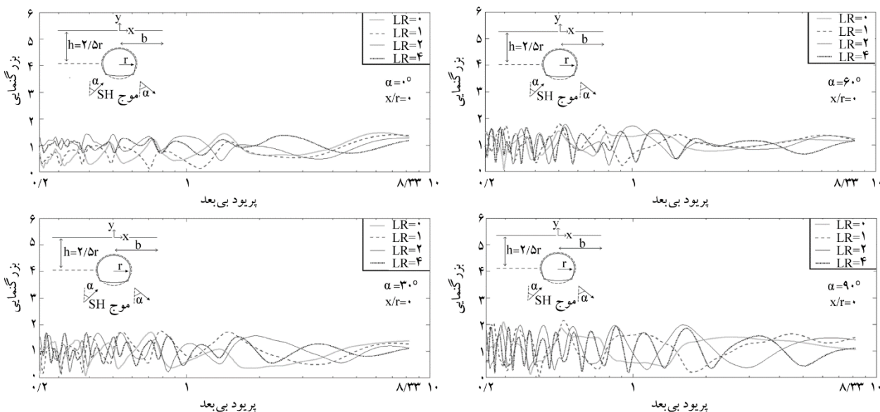
شکل (۱۵): تأثیر نسبت موقعیت افقی بر روی بزرگنمایی سطح زمین بر حسب پرپود بی بعد در نقطه‌ی x/r=0 برای زوایای مختلف موج مهاجم.
